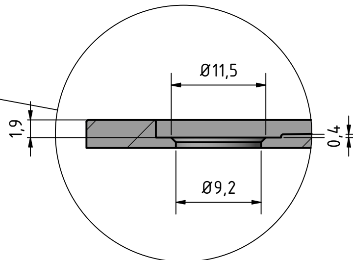
Detalle E
